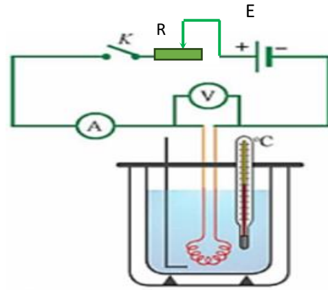
Hình 7: Sơ đồ thí nghiệm đo nhiệt dung riêng
